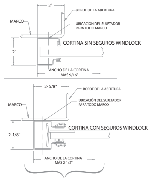
FIGURA 7 SECCIÓN TRANSVERSAL DE LA CORTINA DE LA PUERTA
